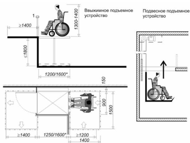
Рисунок 16 – Примеры подъемников различных типов
