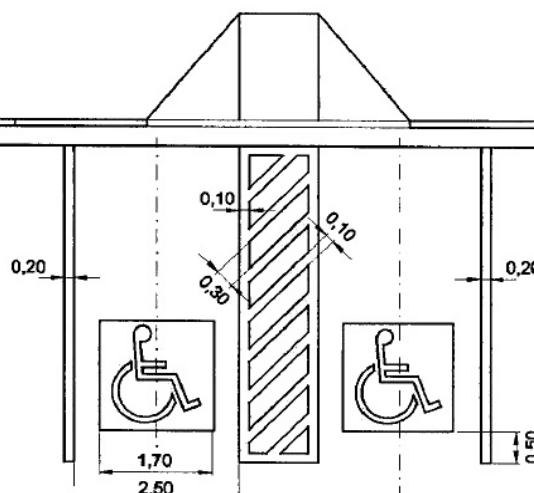
Рисунок Б.2–Типовая схема планировки совмещенных машино-мест для стоянки (парковки) транспортных средств инвалидов перпендикулярно тротуару
